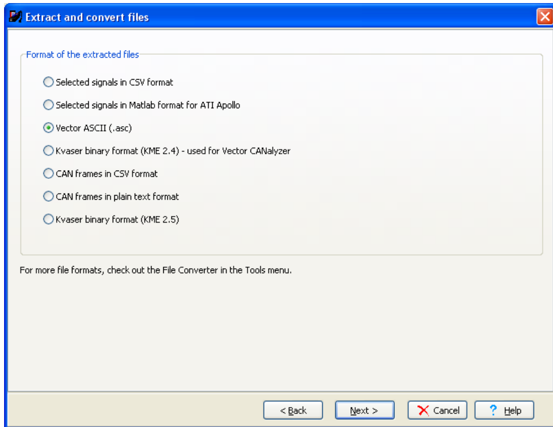
Figure 23. Choose format.
